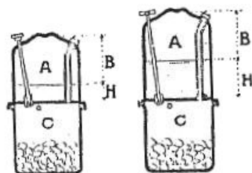
Lampe à réservoir de grande capacité (excès d'eau en fin de marche).
